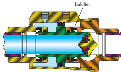
Sperrventil geschlossen
