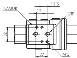
Sperrventil geschlossen
