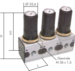
Montagebeispiel für Dreierverkopplung Ausgänge mit verschiedenen Drücken
