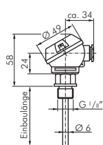
ohne Halsrohr
