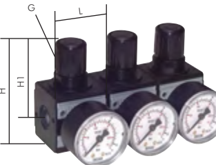
Montagebeispiel für Dreierverkopplung Ausgänge mit verschiedenen Drücken
