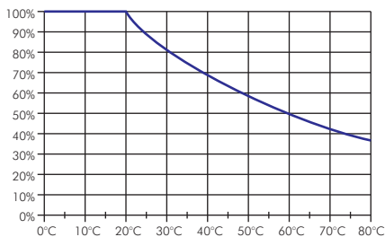
Druck/Temperaturdiagramm PUN-Schläuche
